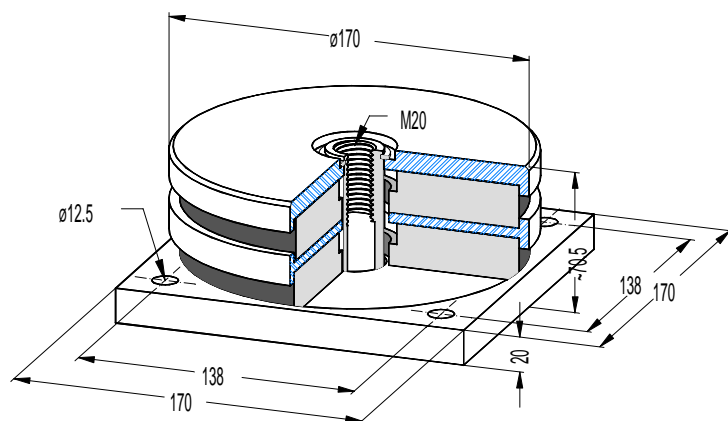
Reihe MF-420 / 520 / 620
