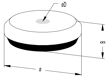
Maschinenfuß Typ T
