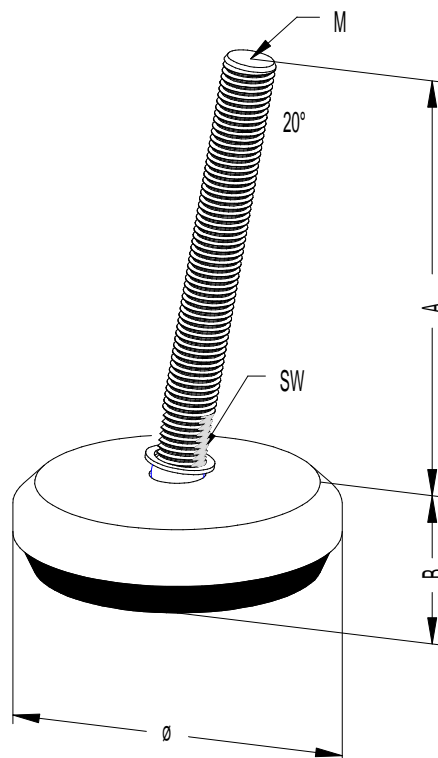
Maschinenfuß Typ K
