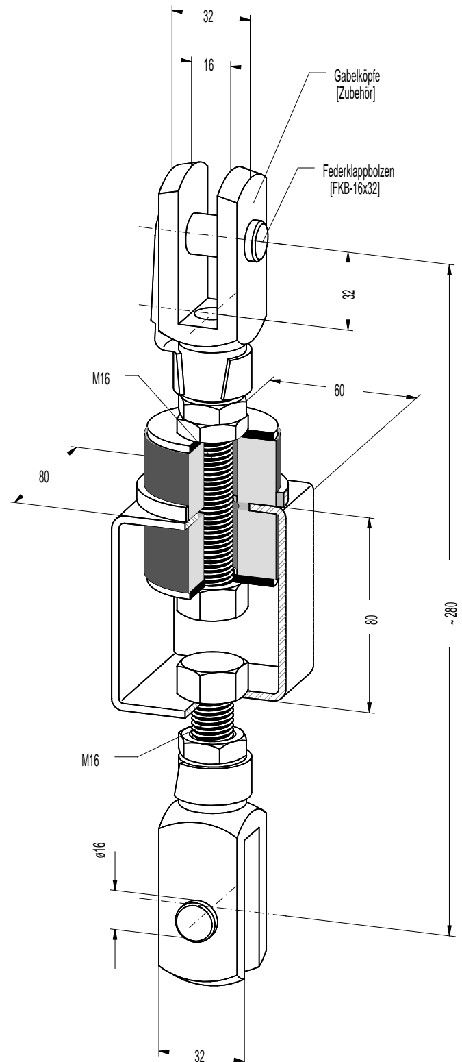
Reihe ADZ-200
