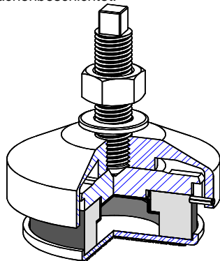
Metaldämpfer mit ABS-Platte
