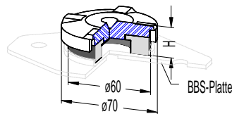
Reihe MD-100
