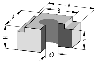
Metallkissen MQL- [ ]
