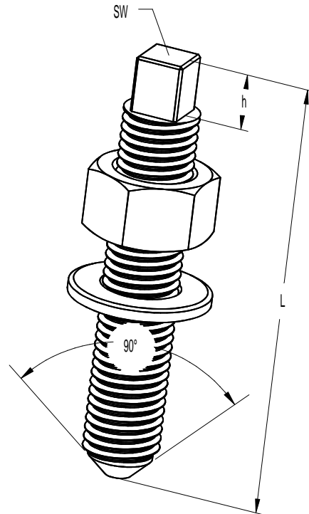
Nivellierschraube NV
