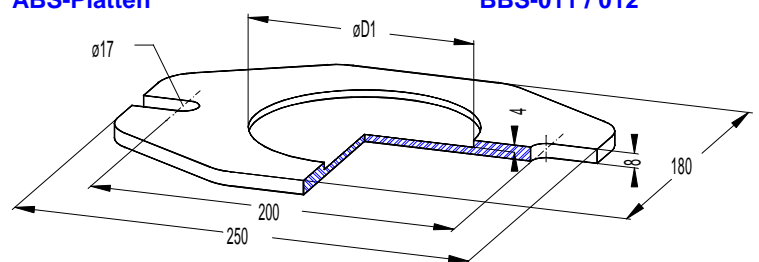
BBS-003 / 004
