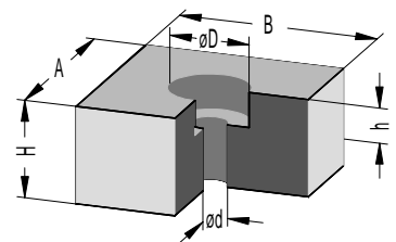
Metallkissen MRA- [ ]
