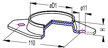
BBS-011 / 012
