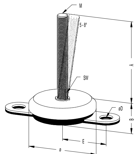
Typ M77
