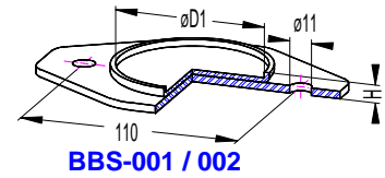
BBS-001 / 002
