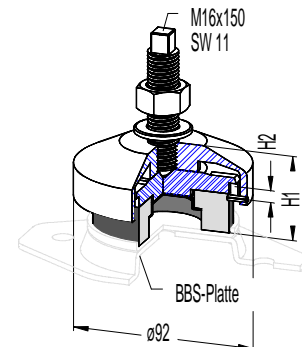
Reihe ND-200
