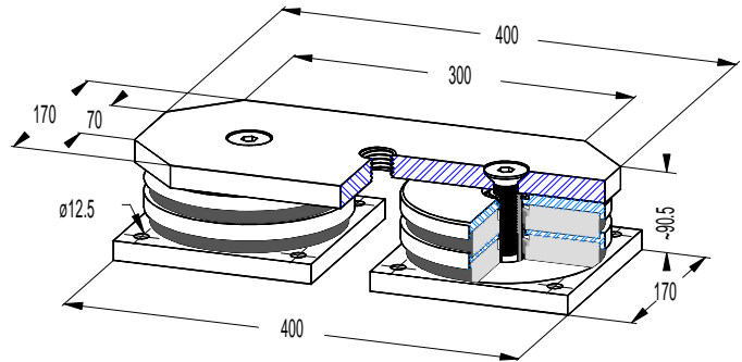
Reihe MF-422 / 522 / 622
