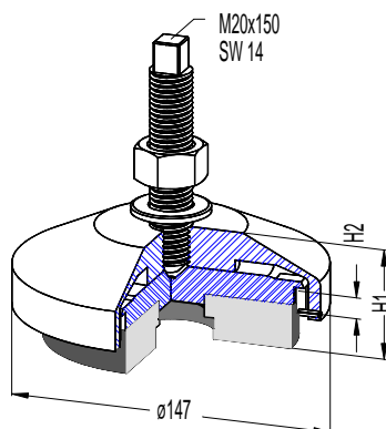
Reihe ND-300
