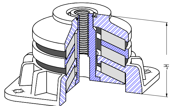
Reihe DZ-420-1 / 520-1
