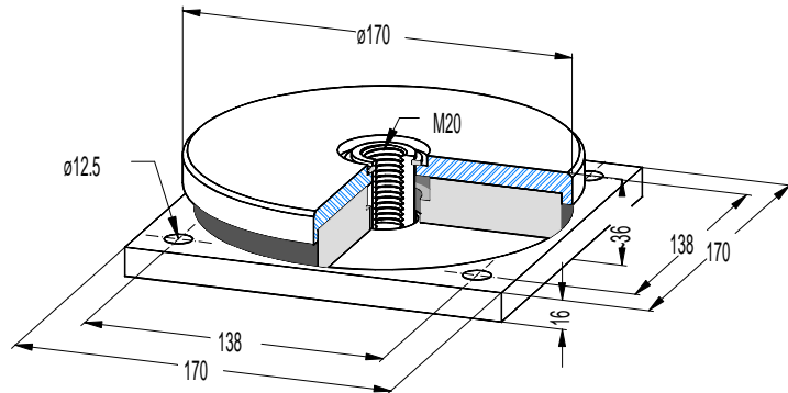
Reihe MF-400 / 500 / 600
