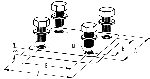
ASP-Platten
