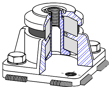
Metaldämpfer mit ASP-Platte
