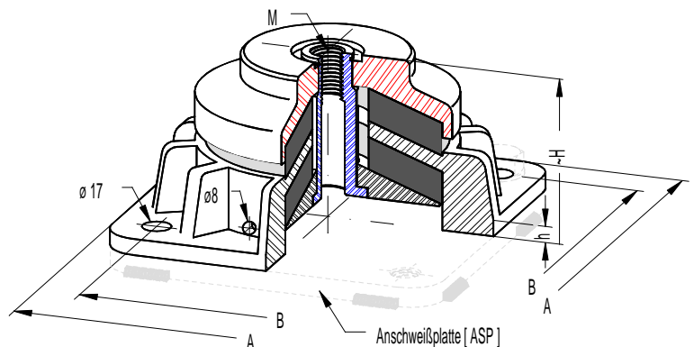
Reihe DZ-400-1 / 500-1
