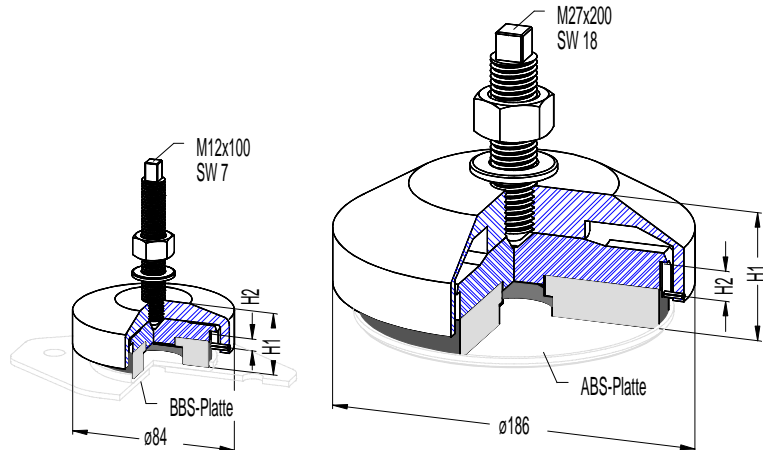
Reihe ND-100
